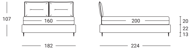
Letto per materasso cm 160x200 Bed for mattress size cm 160x200
