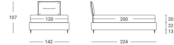
Letto per materasso cm 120x200 Bed for mattress size cm 120x200
